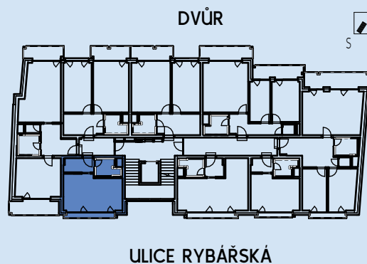
PŮDORYS 5.NP
